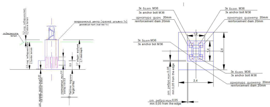
Joonis 4. Vundament HP80□
