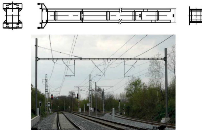
Joonis 8. Põiktala
